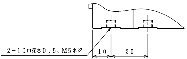
エア-供給口詳細図
