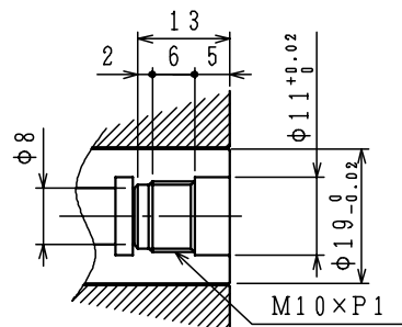
ストッパー (ノズル) 取付け詳細
