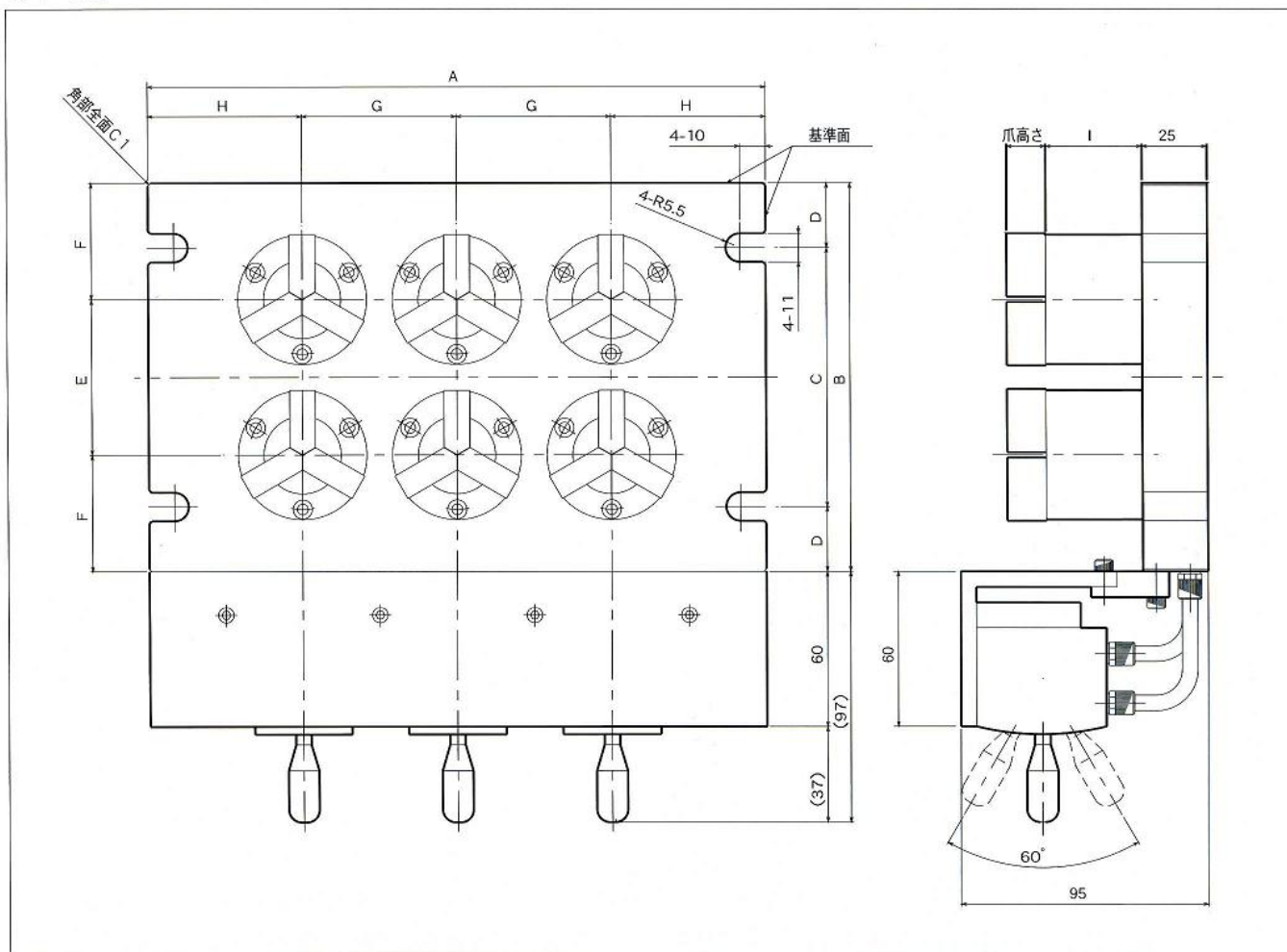
【寸法表】 Dimensions
