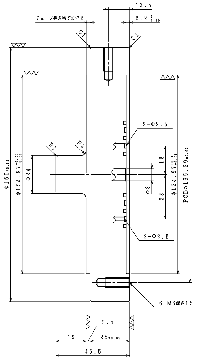
端面部TUVWXYZ断面図
