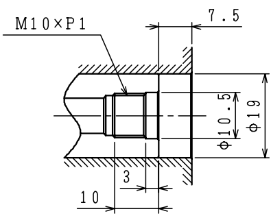
ストッパー (ノズル) 取り付け部詳細
