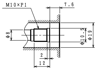
ストッパー（ノズル）取り付け部詳細
