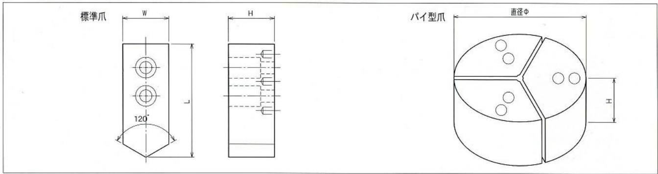
【寸法表】 Dimensions
